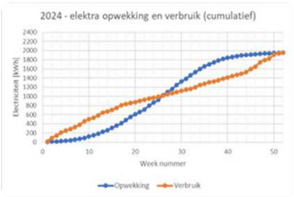
2024: Elektra opwekking (blauw) en verbruik (oranje)
