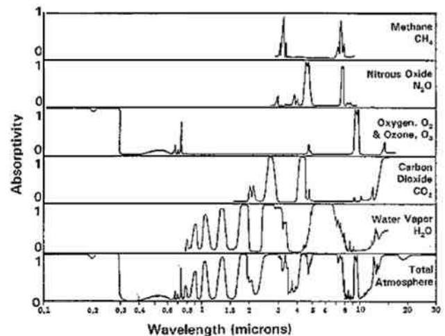
[After J. N. Howard, 1959: Proc. I. R. E. 47 1459; and R. M. Goody G. D. Robinson, 1951: Quart J. Roy. Meteorol. Soc. 77 153]
