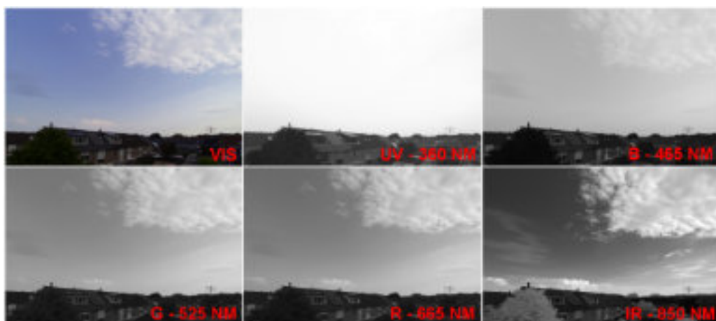
fig 2: Fotoreeks in oplopende golflengten genomen vanuit zolderraam te Maarssenbroek met een UV narrowband filter, daglicht filter uitgesplitst in RGB-kanalen en een IR longpassfilter.
