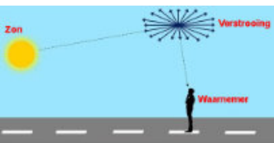
fig 1: Schematisch beeld van Rayleigh verstrooiing in de atmosfeer.
