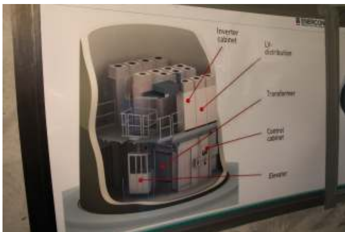
Schema van de apparatuur in de voet van de windmolen
