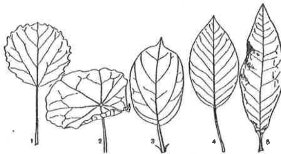
Fig.3. Grootste breedte in het midden. 1 ratelpopulier, 2 O.I. kers, 3 appel (type XI), 4 peer, 5 perzik
