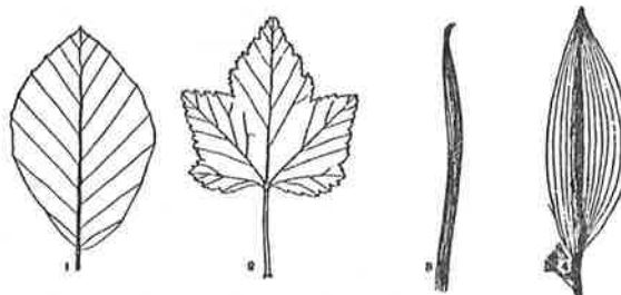
Fig. 2 Nervatuur. 1 Veernervig (beuk), 2 handnervig (bes), 3 en 4 parallelnervig, 3 rechtnervig (gras) 4 kromnervig (lelietje van dalen). Alleen de grotere nerven zijn aangegeven
