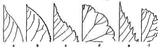
Fig. 7. Kleine insnijdingen. a gaafrandig, sering; b gezaagd, appel; c dubbelgezaagd, iep; d gekarteld, Pelargonium; e getand, tamme kastanje; f gegolfd, ratelpopulier
