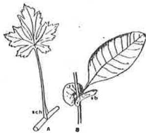
Fig. 1. A. Volledig blad (boterbloem); sch bladschede; B. blad met steunblaadjes (sb) (Jap. kwee)
