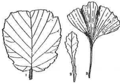
Fig. 5. Grootste breedte boven het midden. 1 Amerikaanse hazelaar, 2 chrysant, 3 Ginkgo
