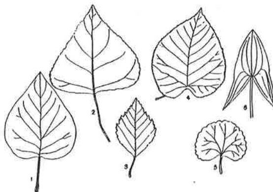
Fig.4. Grootste breedte onder het midden. 1 sering, 2 populier, 3 berk, 4 linde, 5 hondsdrif, 6 pijlkruid
