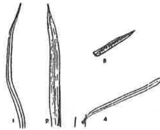
Fig. 6. Breedte overal gelijk. 1 gras, 2 lis, 3 jeneverbes, 4 douglasden
