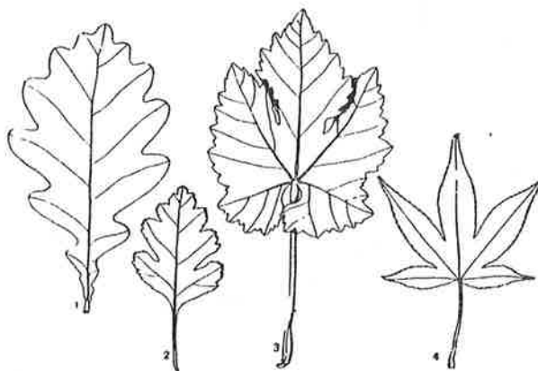
Fig. 8. Diepere insnijdingen. 1 eik, veerlobbig, 2 meidoorn, veerspletig, 3 druif, handspletig, 4 jap. esdoorn, handdelig
