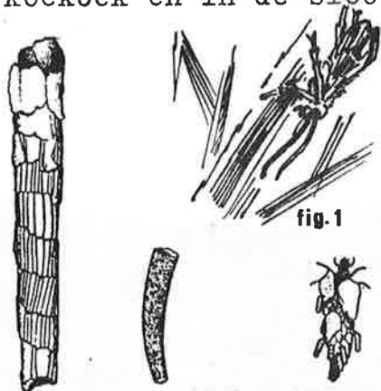
fig.2 Kokertjes van de kokerwormen
