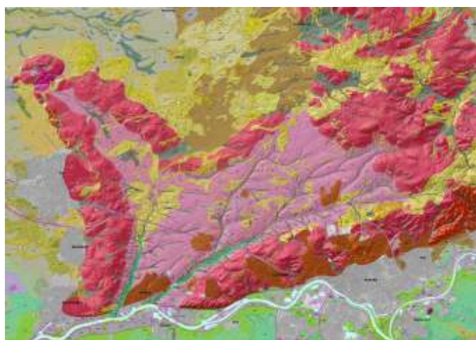
fig.2 Geomorfologische kaart van de stuwwallen
