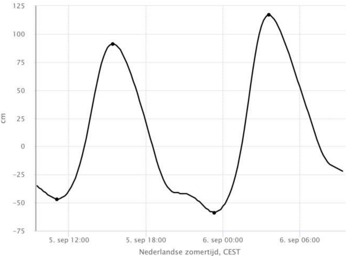
Afb.: Scheveningen - Rijkswaterstaat Waterinfo, Waterhoogte Astronomisch t.o.v. NAP
